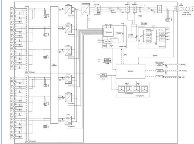
电路框图
